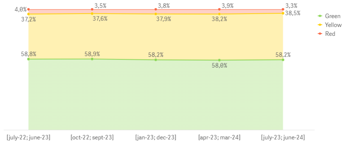
PIGS - Sows
