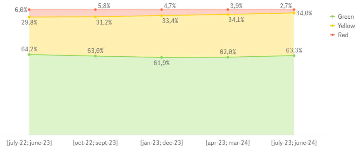
PIGS - Sows
